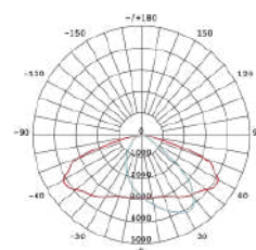
CURVA TII-M
